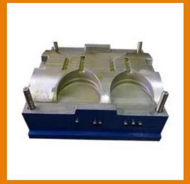
Dustpan Mould Die
